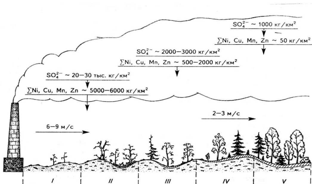
Рис. 1. Зоны деградации экосистем северной тайги: I – «техногенная пустошь»; II – промышленно-техногенная березово-криволесная лесотундра; III – существенно разрушенные экосистемы; IV – начальная стадия деградации экосистем; V – самая начальная стадия деградации экосистем
